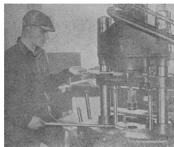
図1.可塑性の金属は溶解釜から取鍋に掬い取り、ダイカスト機の圧縮室へと移される
