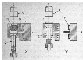
図2.可塑性の銅合金よりダイカストを圧縮するPolak機の働きを示すダイヤグラム
