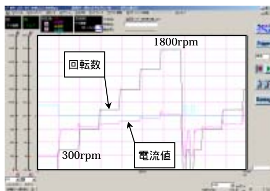
図2 サーボモータ回転数制御
