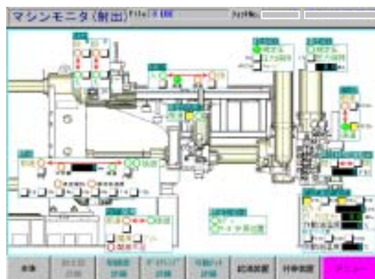
図1 マシンモニタ画面(射出ユニット)
