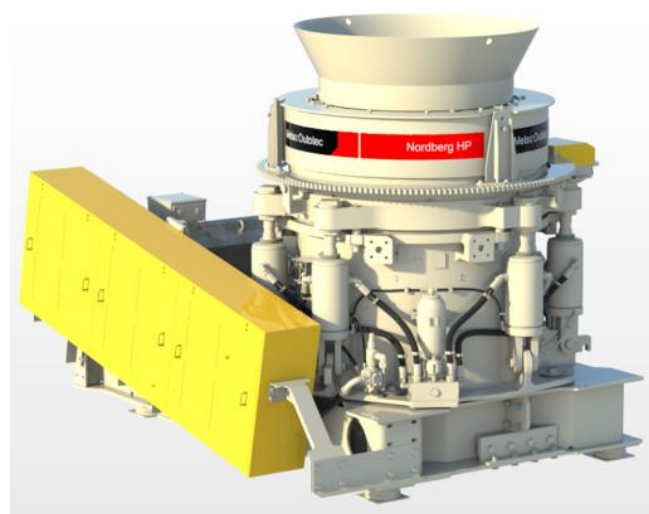
図一 2 HP 5 外形図
