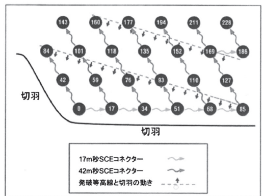
図2 a：2.8m×3.2mパターン-時間は17m秒と42m秒の遅延
