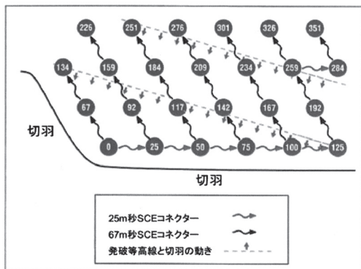
図2 b : 4.4m × 4.7mパターン-時間は25m秒と67m秒の遅延 この発破により、発破行穴間のスピードは5.3m秒/mで、発破列穴間のスピードは、14.9m秒/mとなります。
