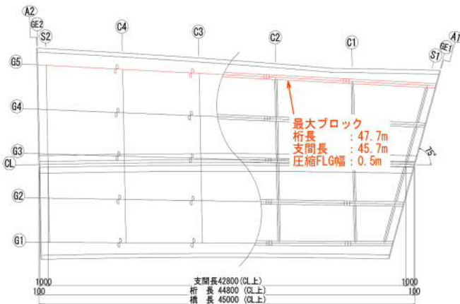
図-1 橋梁平面図
