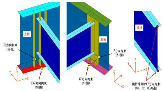
図-4 拘束条件
