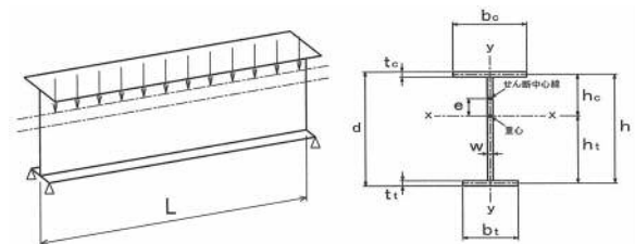
図-2 単純支持の I 形断面部材
