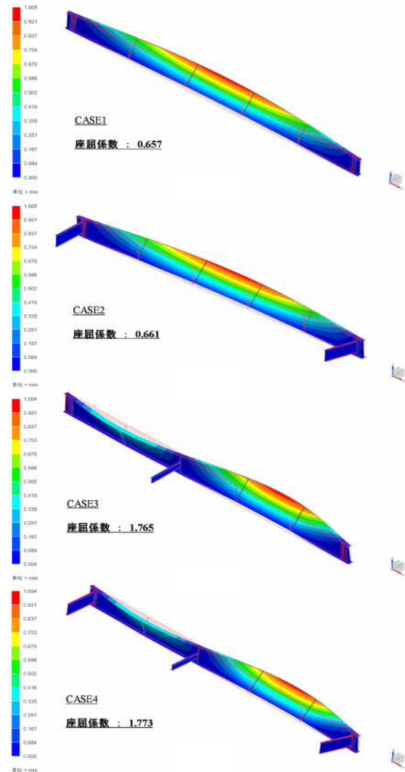
図-5 解析結果
