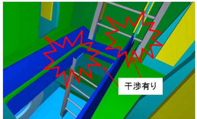
図3 干渉チェック (梯子とリブの干渉)
