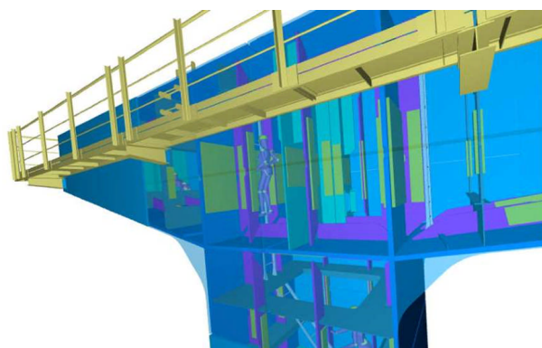
図 2 詳細度 300 モデル例 (鋼製橋脚)
